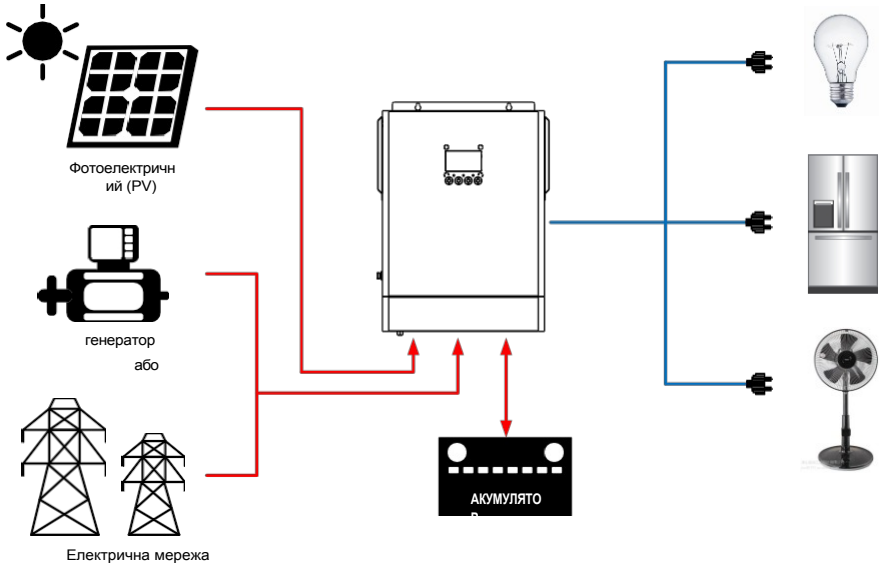
Схема системи
